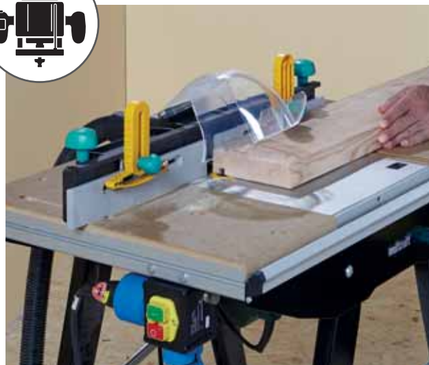
Maróasztal
