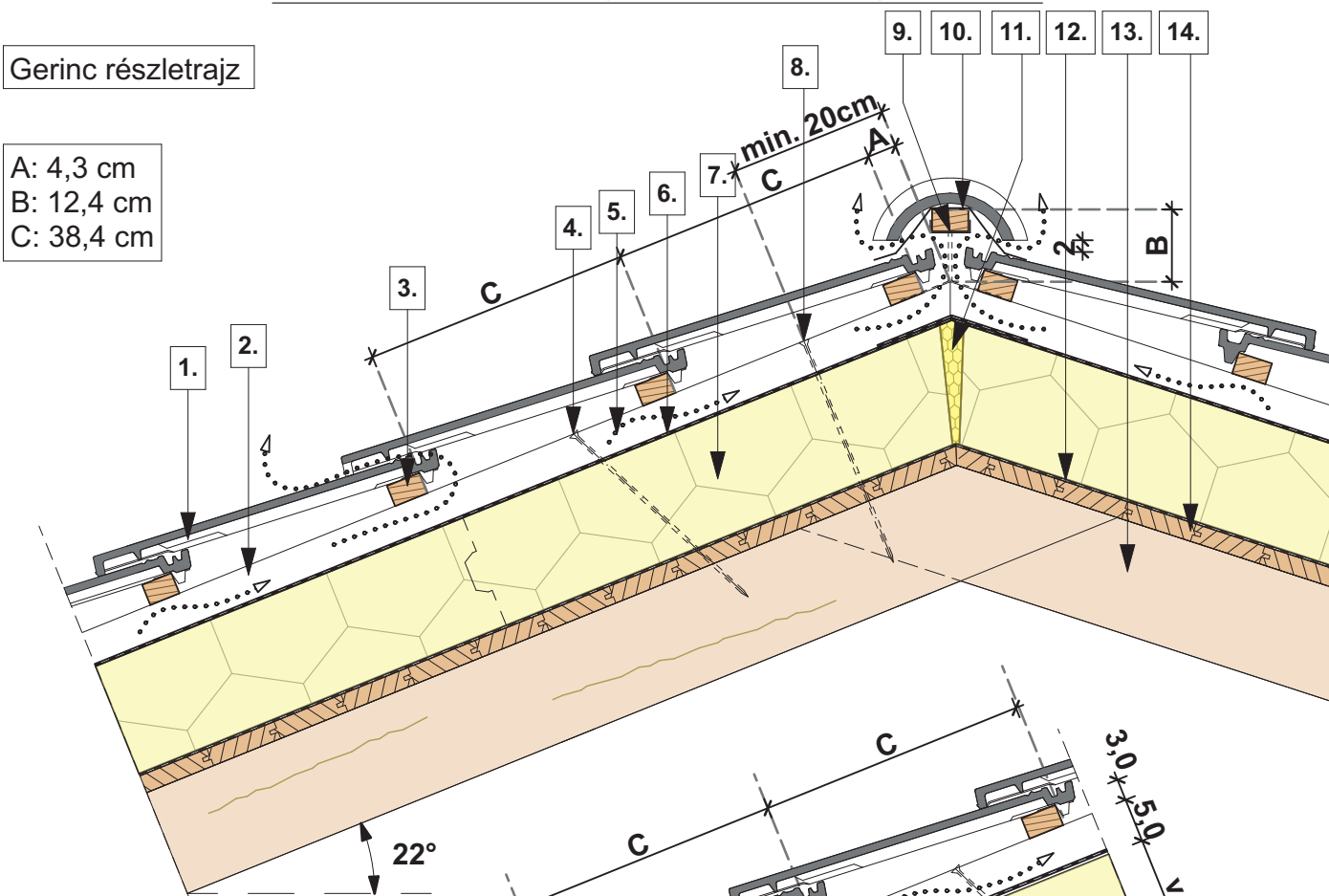
Eresz részletrajz
