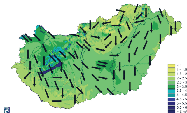
Magyarország jellemző szélirányai országos területi elosztásban
