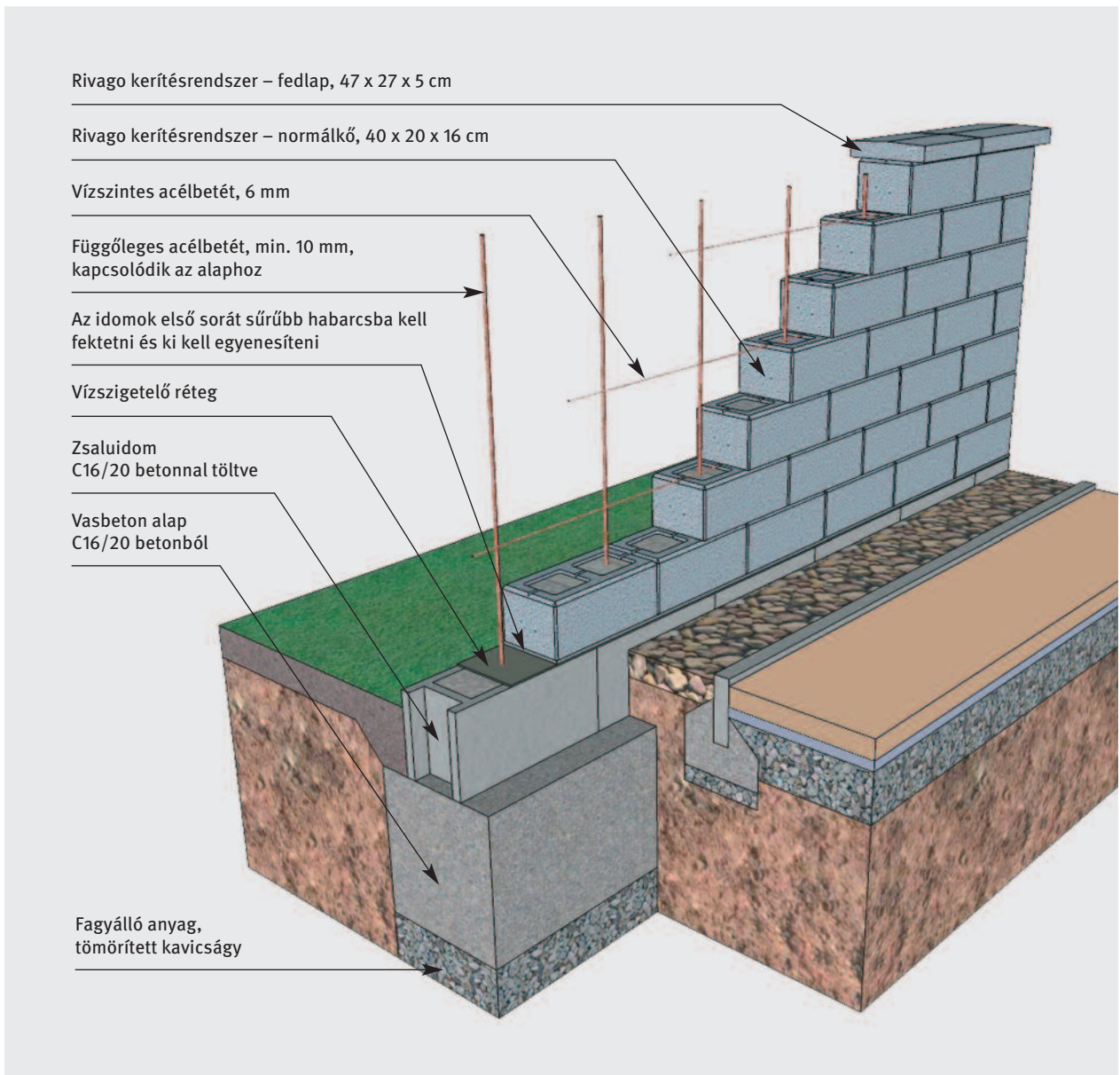
Rivago idomokból készült kerítés metszetének perspektivikus nézete
