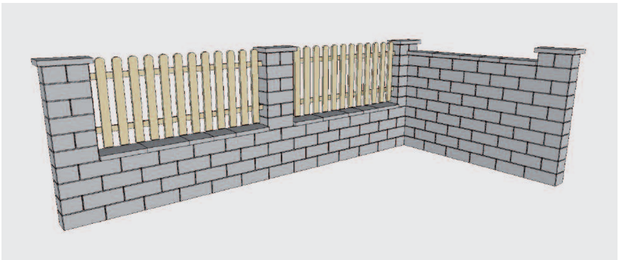
Rivago idomokból készült kerítés és 40 x 20 cm méretű oszlopok lehetséges megoldásának perspektivikus nézete
