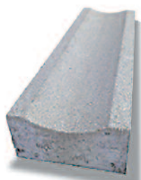
Betonfolyóka 2,5 cm horonymélységgel Méret: 50 x 20 x 8 cm
