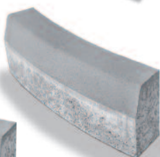
Íves útszegélyek Méretek: 78 x 25 x 15 cm, R = 3,0 m 78 x 25 x 15 cm, R = 2,0 m 52 x 25 x 15 cm, R = 1,0 m 39 x 25 x 15 cm, R = 0,5 m
