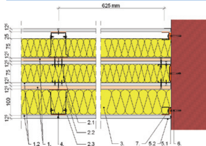
Fal 6 CW 75/125 + 2 előtétfal CD profilvázon
