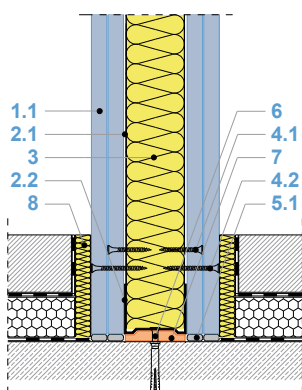
Szerelt fal lábazati csatlakozása nyers földmehhez
