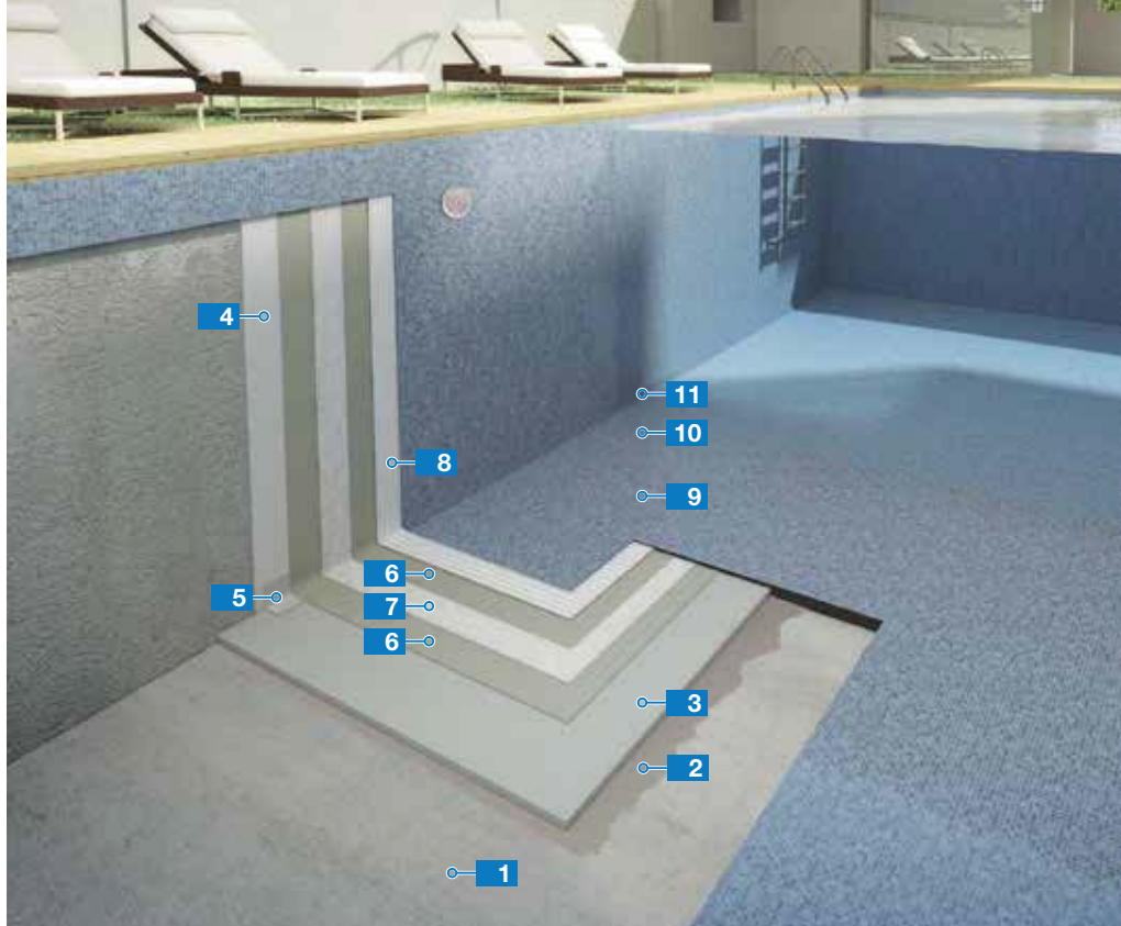
Vízszigetelő rendszer üvegmozaik fektetéséhez úszómedencében
