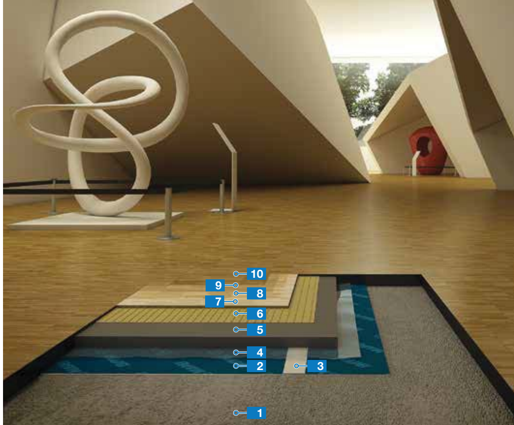
Ultragyors hangszigetelő rendszer mozaik parkettához
