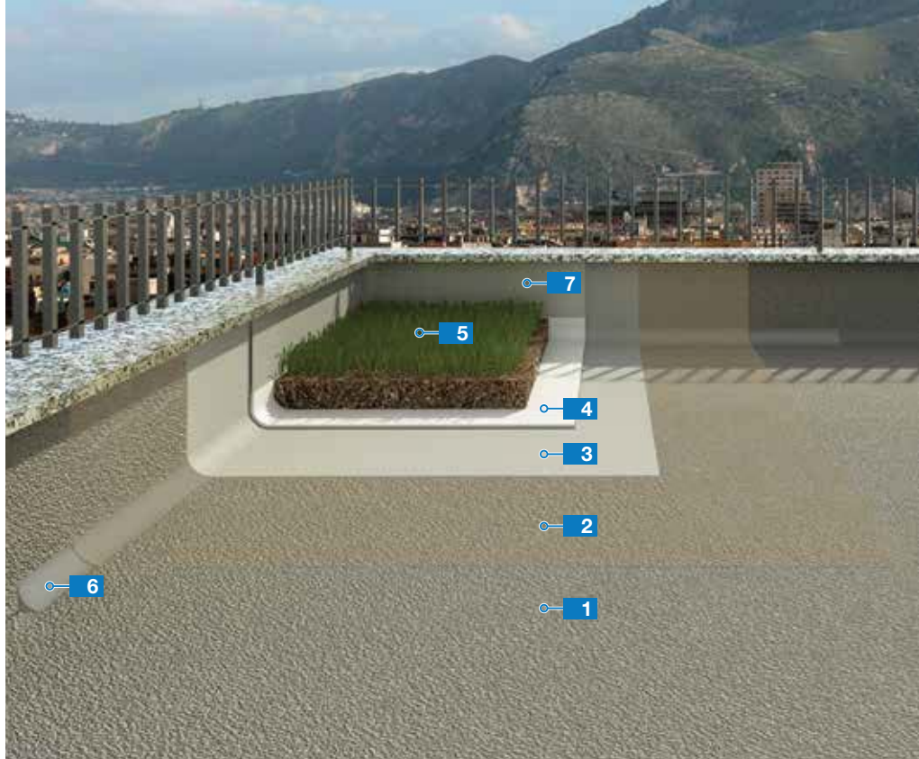
Szórt hibrid poliurea vízszigetelés zöldtetőhöz
