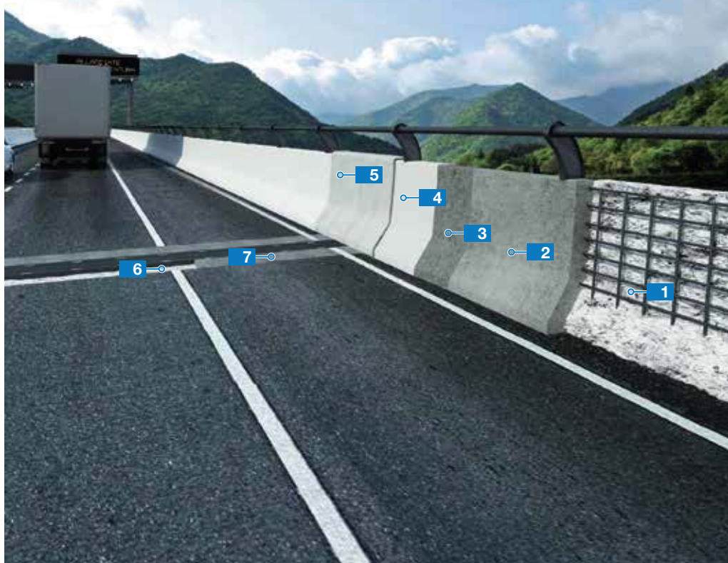
Vasbeton korlátok javítása és csatlakozások autópályán
