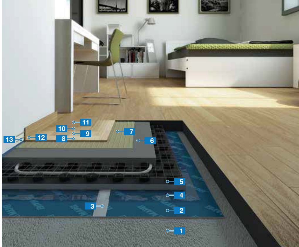
Hangszigetelő rendszer fapadló fektetéséhez fűtött esztrichen
