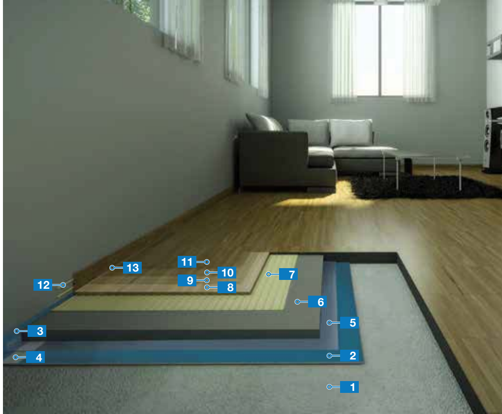
Gyors hangszigetelő rendszer fapadló fektetéséhez
