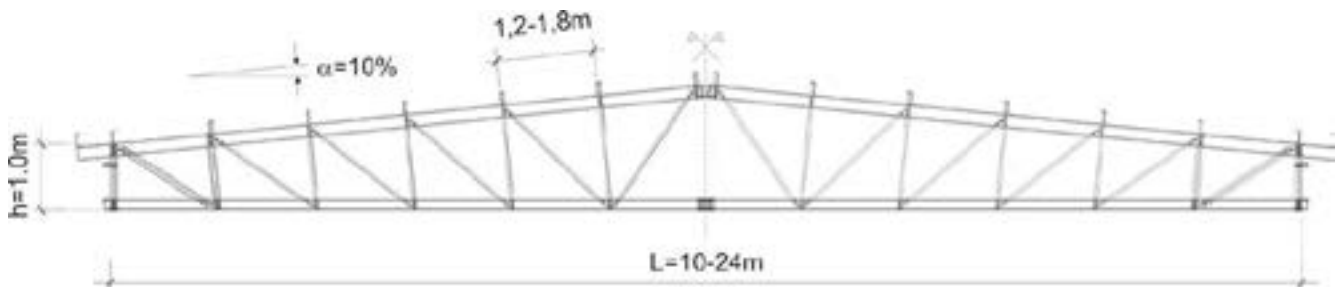
5. ábra. Kéttámaszú típusstartó
