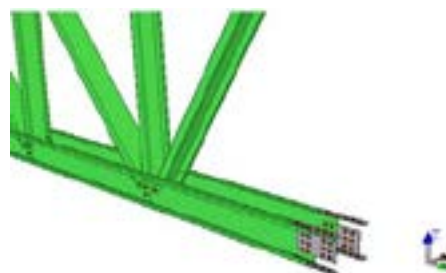
4. ábra. Felső és alsó övrúd helyszíni illesztése
