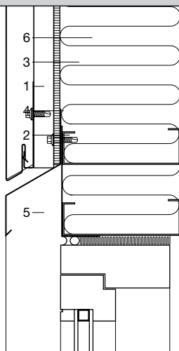
Ablak felső csomópontja – függőleges metszet
