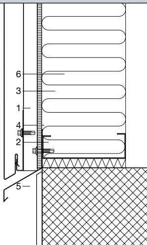
Lábazati csomópont – függőleges metszet
