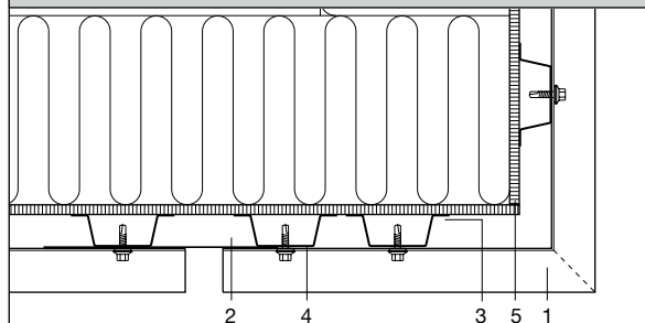
Sarokmegoldás – vízszintes metszet
