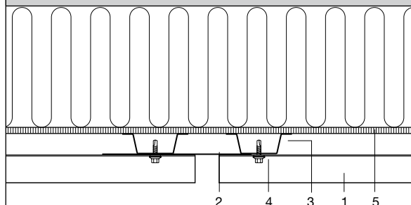
Függőleges hézag – vízszintes metszet
