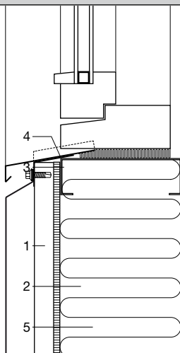
Ablak alsó csomópontja – függőleges metszet
