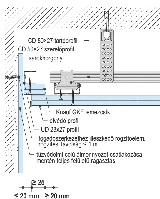
D113 - Mozgási hézag tűzvédelmi kivitelben
