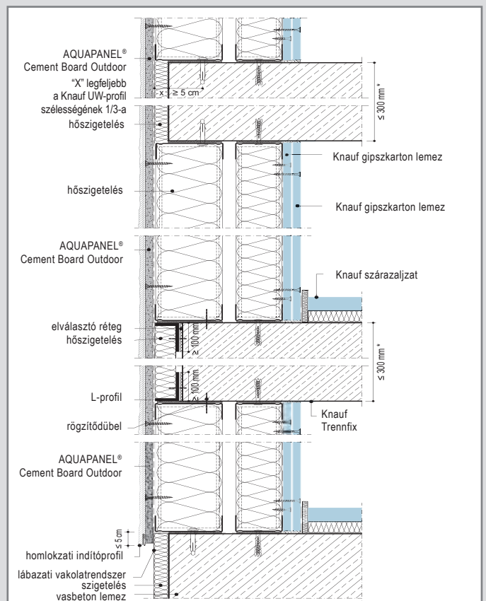
W388E-V1 Metszet
