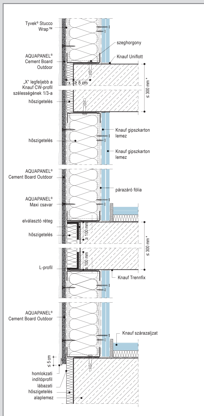
W 384E-V2 Metszet-2
