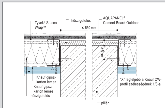
W384E-HS1 Falhoz vagy betonpillérhez csatlakozás
