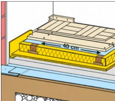
1 Faszerkezetű padló: 10 cm ISOVER QUATTRO ISOVER TDPT 20/20
