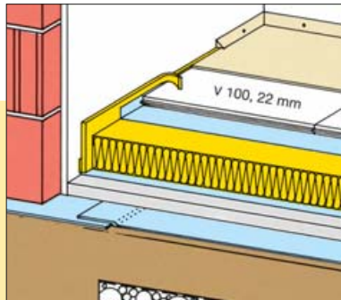
3 Fa építőlemez szárás burkolat *kétrétegű, ragasztott, csavarozott ISOVER TDPT 60/60
