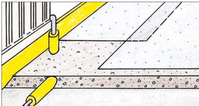
Az ISOVER kerületi szegélyszalvét a feltöltés tetejéig is el lehet helyezni.
