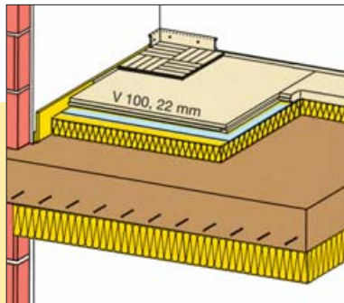
3 Száras burkolat: ISOVER TDPT 50/50, 6 cm ISOVER KDP vagy 12 cm ISOVER KDP
