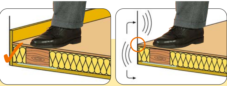
Helyes: A padlószerkezetet az ISOVER kerületi szegélyszávvál el kell választani a faltól.
