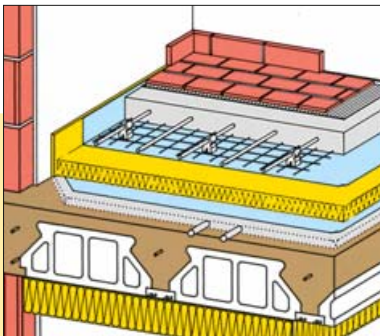
2 Úsztatott esztrich: ISOVER TDPT 50/50, 6 cm ISOVER KDP vagy 12 cm ISOVER KDP
