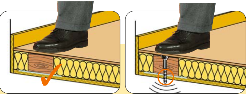
Helyes: A párnafákat a csúsztató polietilén fóliára szabadon kell fektetni.
