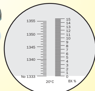
Kalibrált fénytörési skála
