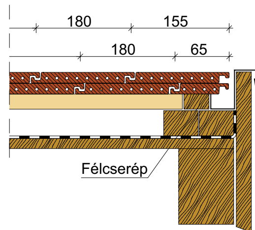
Jobb oromszegély, félcseréppel
