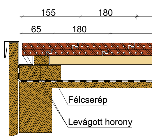
Bal oromszegély, félcseréppel
