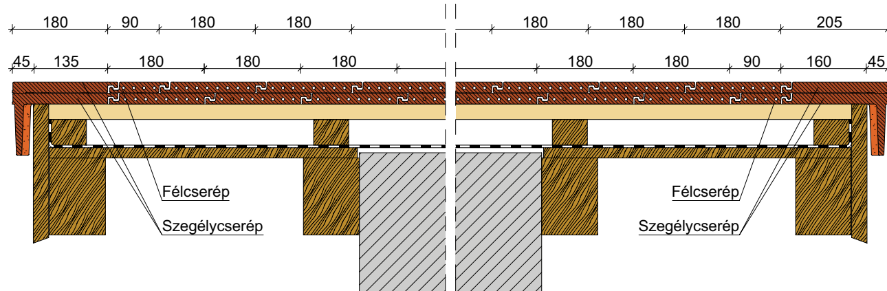
Oromszegély, szegélycseréppel és félcseréppel
