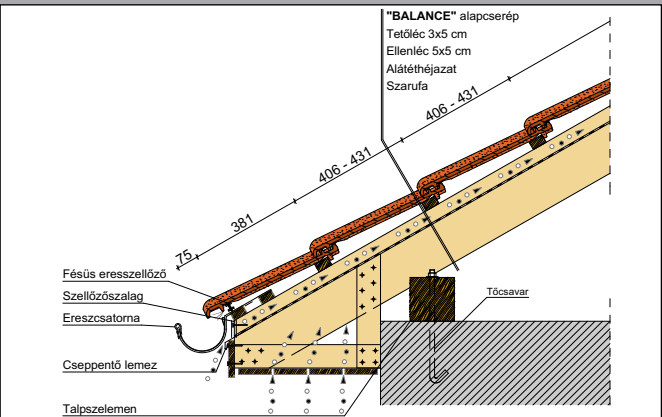
Dobozolt eresz kialakítás
