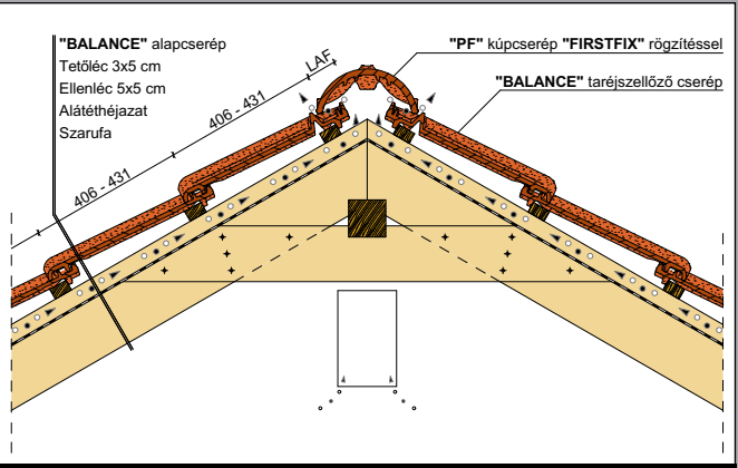
Gerinc kialakítás, taréjszellőző cseréppel
