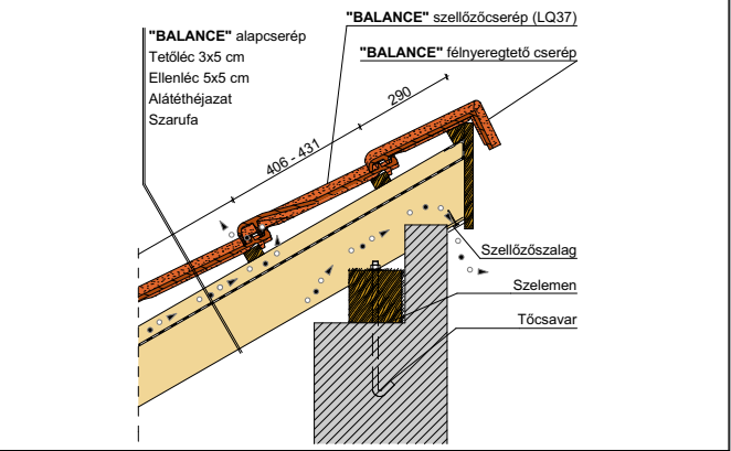
Félnyeregű gerinc kialakítás
