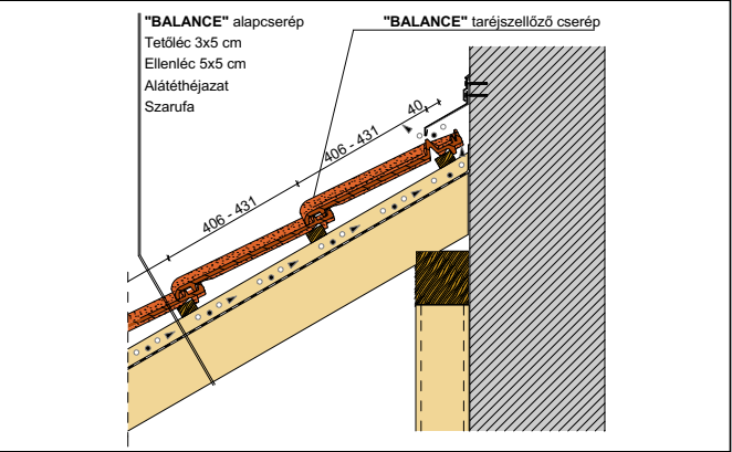
Falszegély kialakítás
