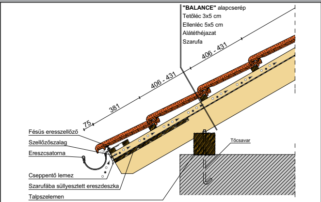
Eresz kialakítás
