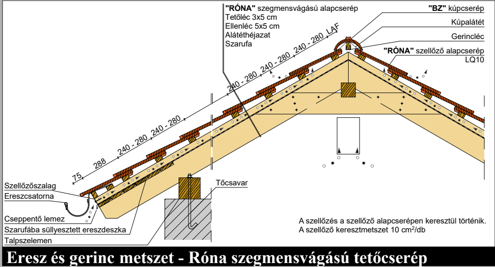
Eresz és gerinc metszet - Róna szegmensvágású tetőcserép
