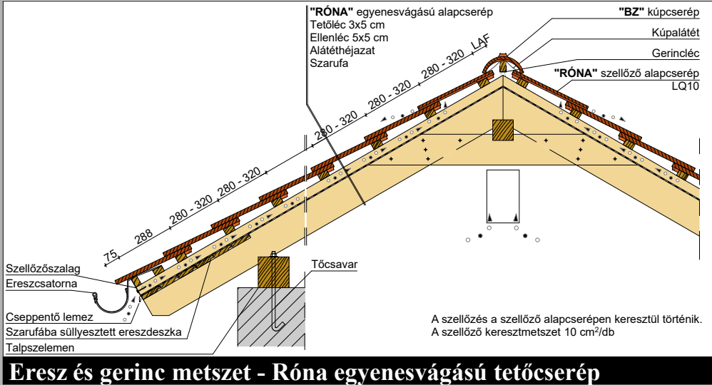
Eresz és gerinc metszet - Róna egyenesvágású tetőcserép
