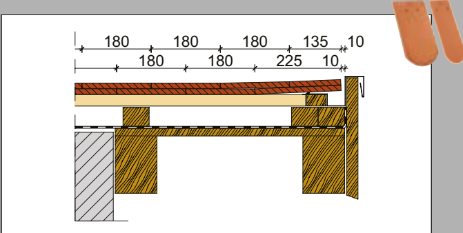
Oromszegély 3/4 és 5/4 hódfarkú cserepekkel
