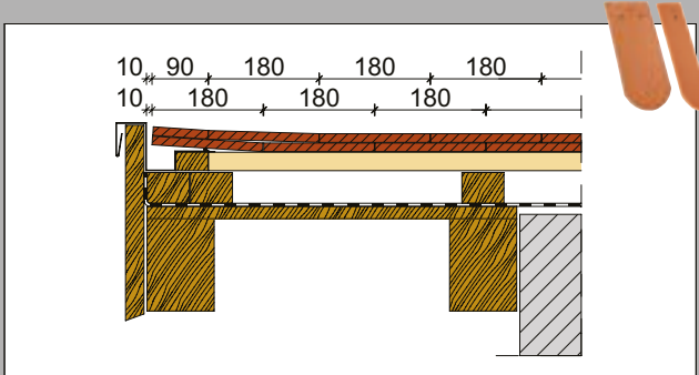
Oromszegély 1/2 és 1/1 hódfarkú cserepekkel
