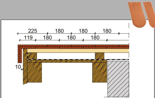
Oromszegély 3/4 és 5/4 szegélycserepekkel
