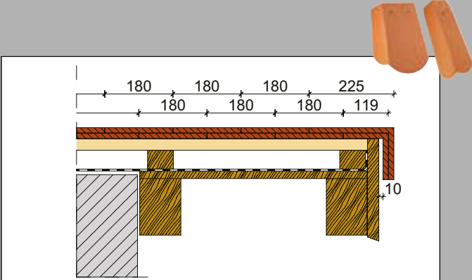
Oromszegély 3/4 és 5/4 szegélycserepekkel
