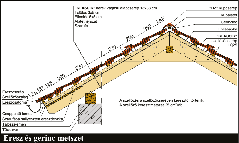
Eresz és gerinc metszet
