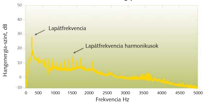
Példa a ventilátor hangspektrumára
