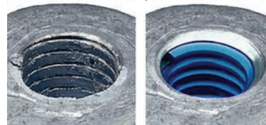
roncsolódott menet javított menet
